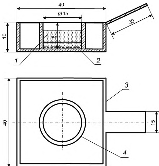
Рисунок 11.2 — Стандартный образец
