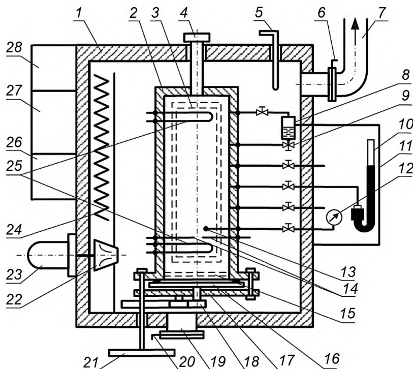
1 — термощаф; 2 — реакционный сосуд; 3 — смотровое окно; 4 — продувочный патрубок; 5 — термоэлектропреобразователь блока регулирования температуры; 6 — задвижка; 7 — вентиляционный патрубок; 8 — испаритель; 9 — вентиль; 10 — ртутный манометр; 11 — пневмопульт; 12 — газовый термометр; 13 — датчик термометра; 14 — электроды источника зажигания; 15 — огнепреградитель; 16 — нижняя крышка; 17 — коромысло; 18 — шестерни; 19 — продувочное отверстие; 20 — заслонка; 21 — штурвал; 22 — вентилятор; 23 — электродвигатель; 24 — электронагреватели; 25 — перемешиватели; 26 — источник зажигания; 27 — электропульт; 28 — блок регулирования температуры
