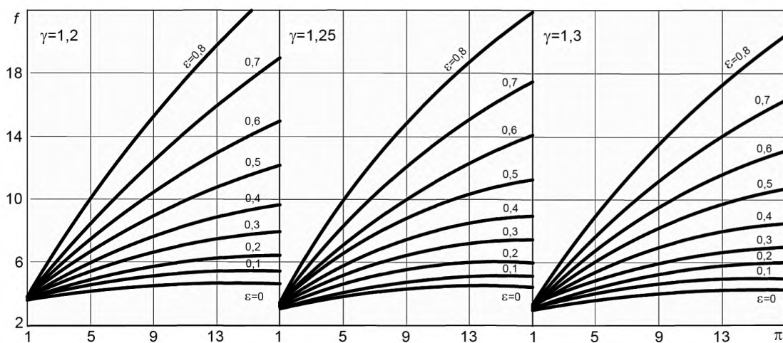
Рисунок П.8.1, лист 1 — Номограммы зависимости функции f(\pi_e, \gamma_u, \varepsilon) от параметров \pi_e , \gamma_u , \varepsilon
