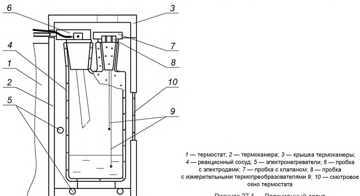
Рисунок 27.1 — Реакционный сосуд
