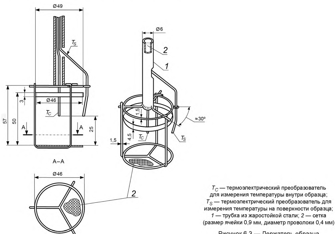
Рисунок 6.3 — Держатель образца
