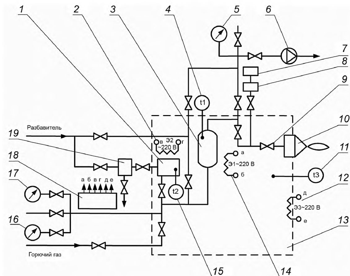
1 — парогенератор; 2 — нагреватель Э2; 3 — ресивер; 4 — первичный термопреобразователь t_1 ; 5 — вакуумметр; 6 — вакуумный насос; 7 — измерительное устройство сигналов с датчика давления; 8 — датчик давления; 9 — вентиль точной регулировки; 10 — насадок диффузионного горения; 11 — первичный термопреобразователь t_3 ; 12 — нагреватель Э3; 13 — термостат; 14 — нагреватель Э1; 15 — первичный термопреобразователь t_2 ; 16 — вакуумметр; 17 — манометр; 18 — система терморегулирования; 19 — емкость для воды
